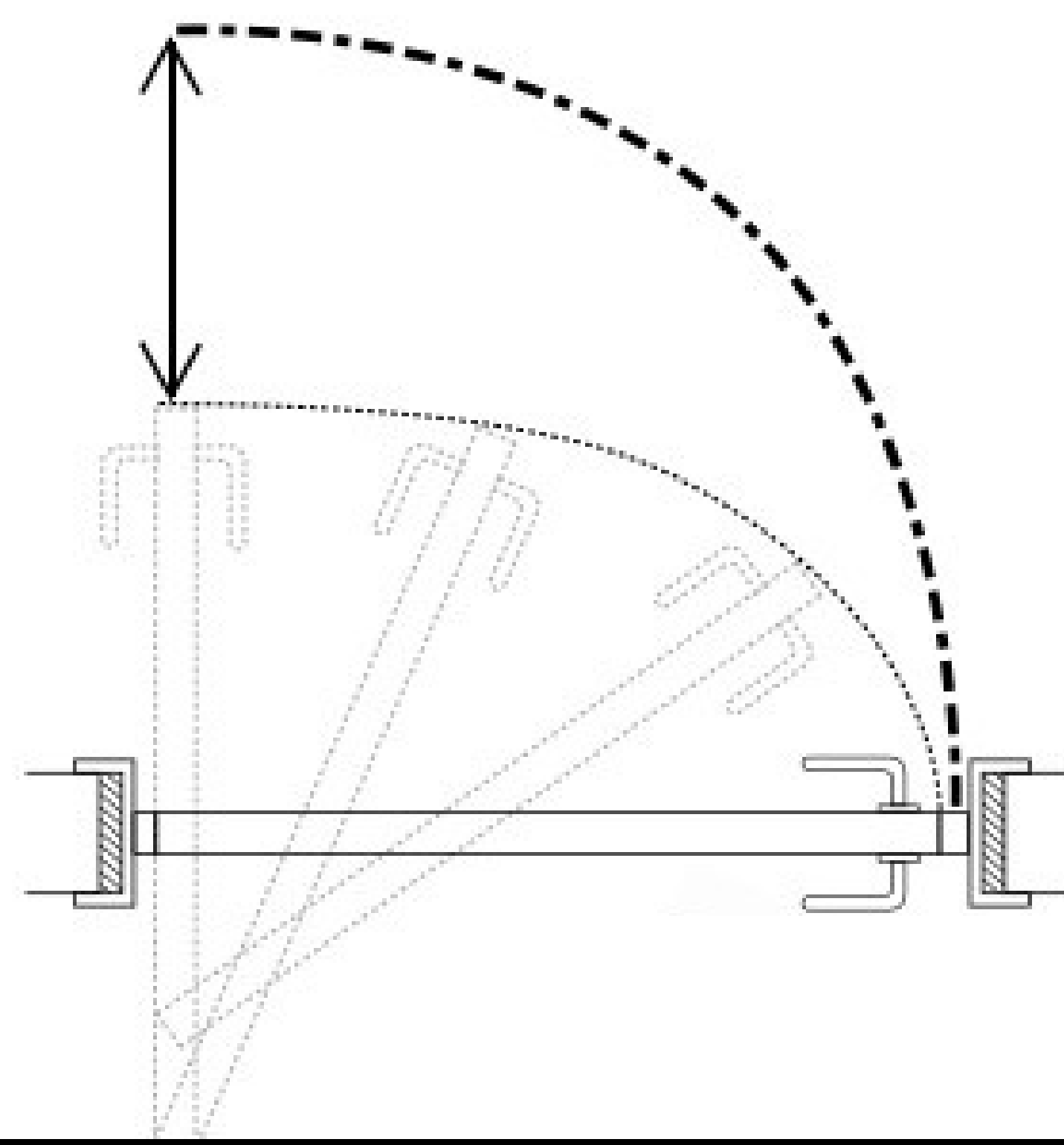
PORTA ROTOTRASLANTE
